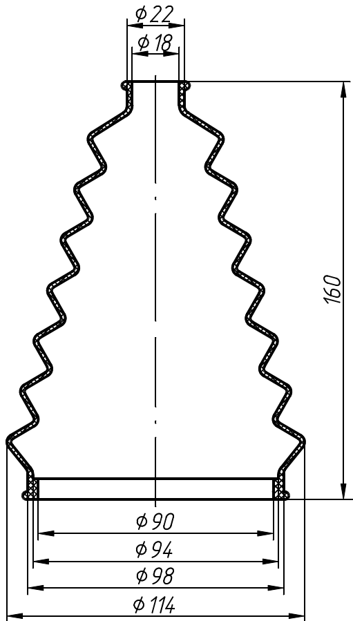
ЯИУМ.РТИ.476 Чехол защитный
