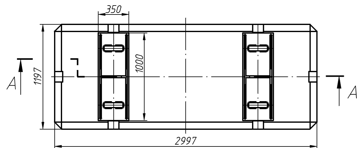
Рабочая накладка 0280/0183
