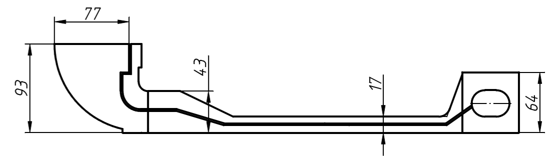
P1481.00.00 Дюбель
