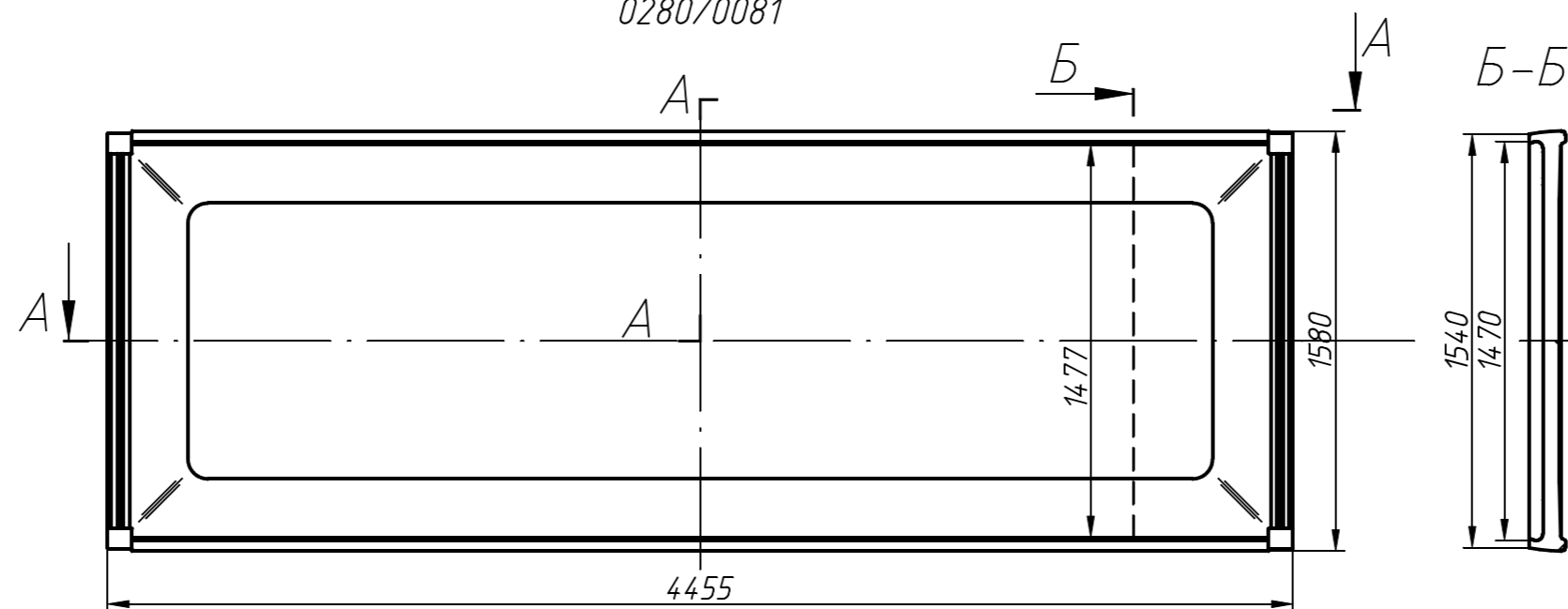
Рабочая диафрагма 0280/0081
