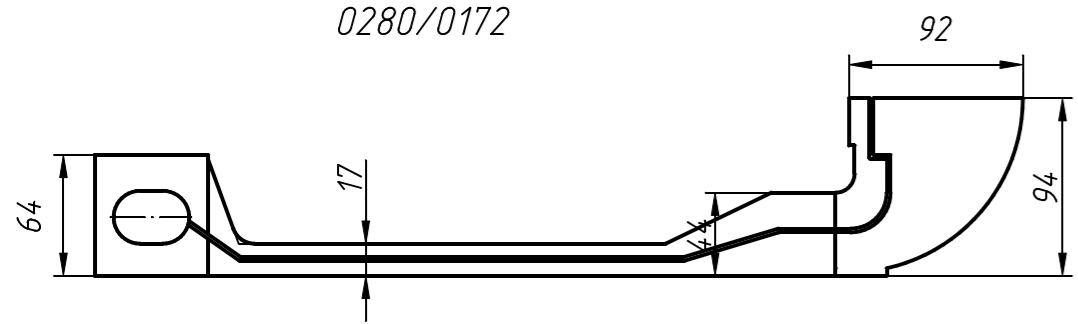
Дюбель 0280/0172
