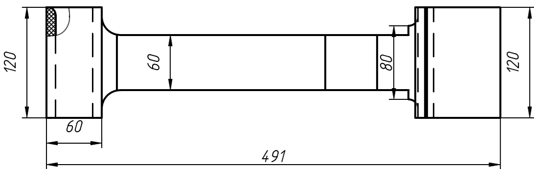
Наполнитель контейнера 0280/0169
