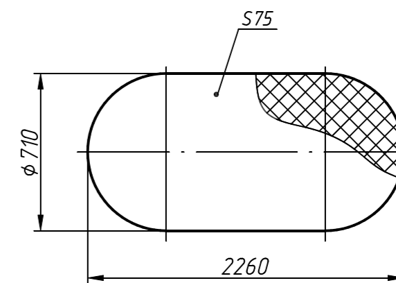
Подушка ЯО 6017.019.807
